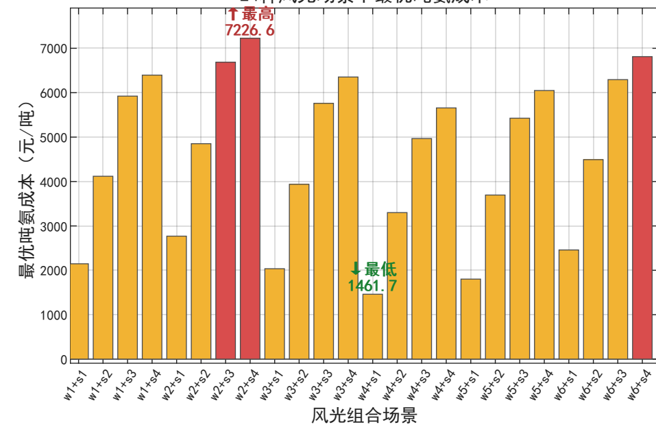
24种风光场景下最优吨氨成本
